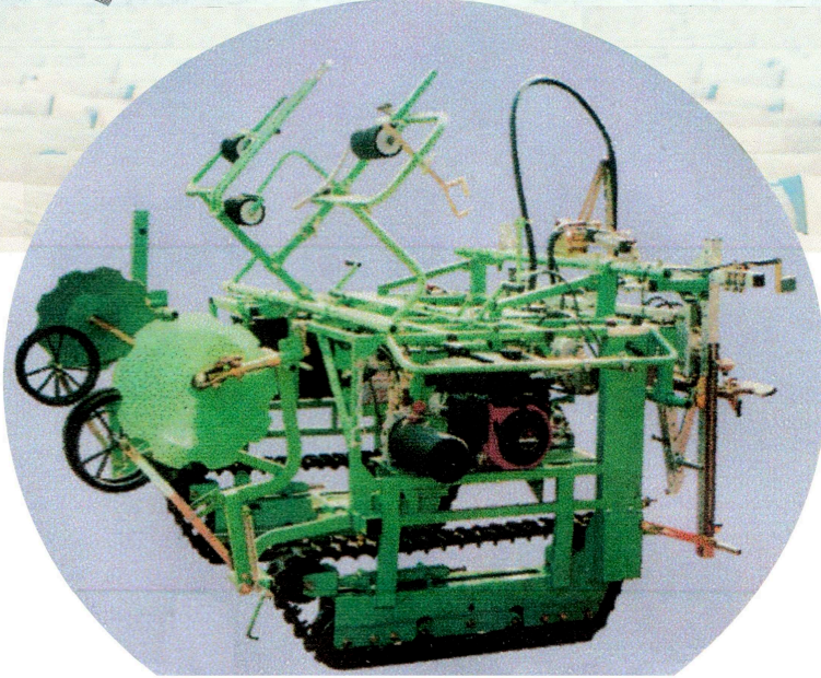
上図 ゴムクローラータイプ PS2-C-135DC-OP (往復タイプ)
